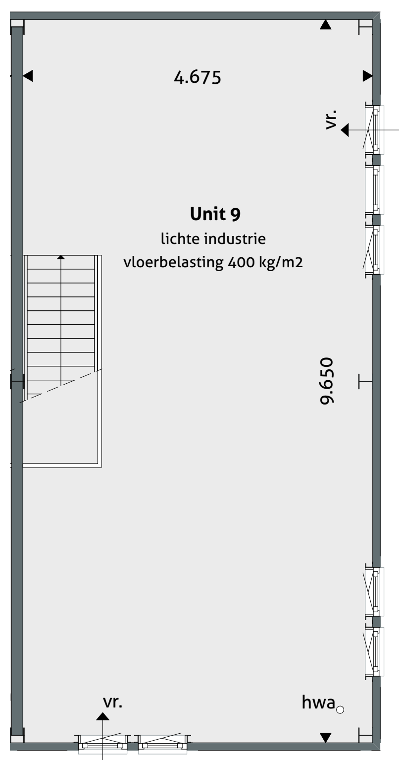
Verdieping 1:100
