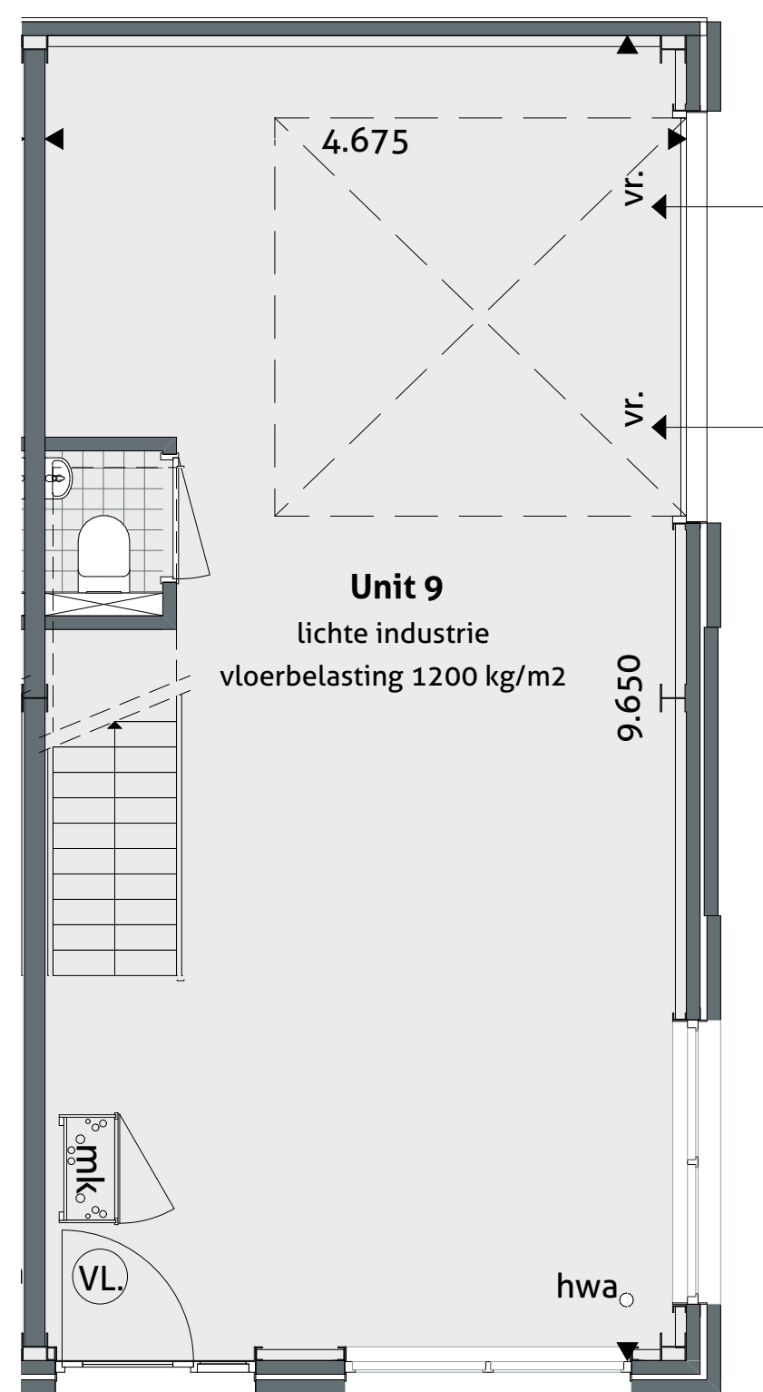
Begane grond 1:100
