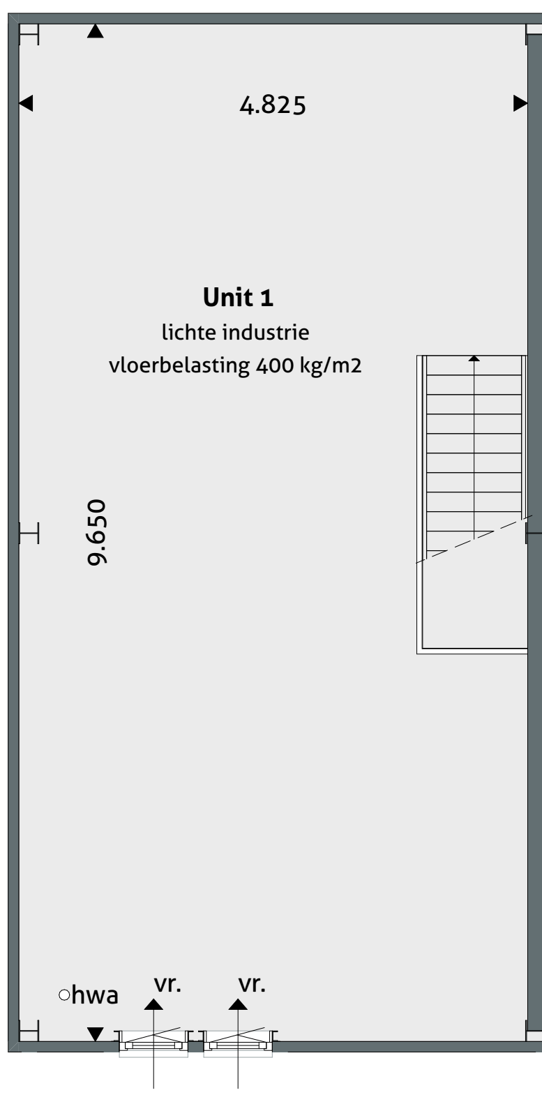
Verdieping 1:100
