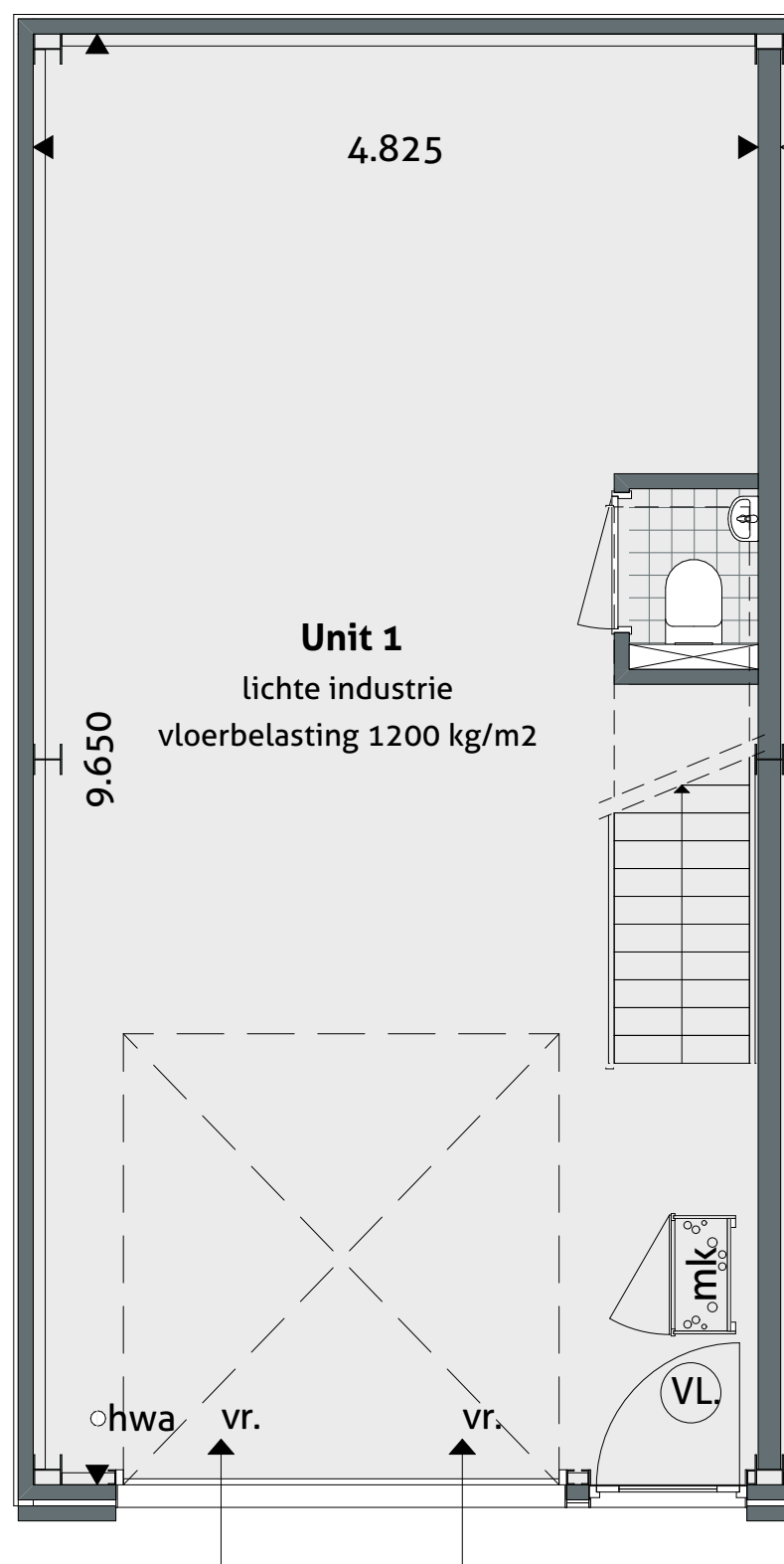
Begane grond 1:100
